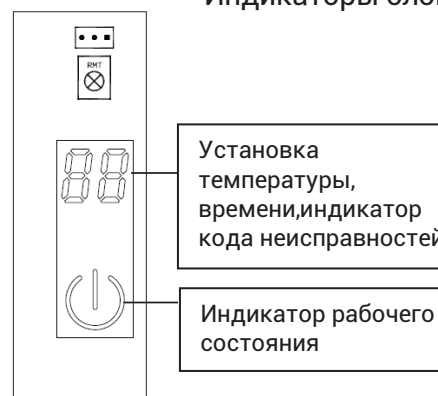
Индикаторы блока 22
