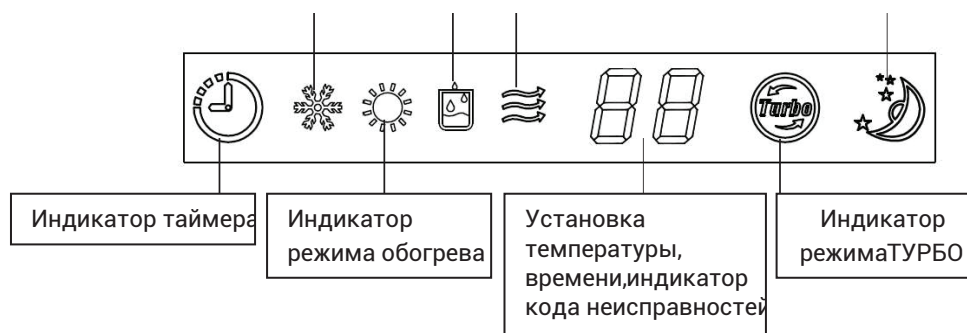
Индикаторы блока 19
